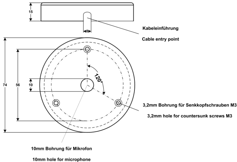
Skizze Montageflansch
